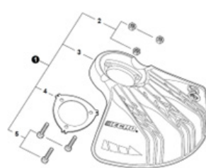
Protector para cuchilla
